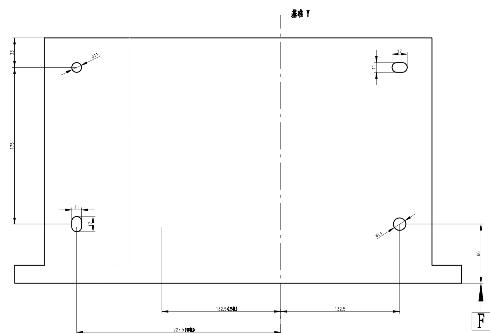
底面外形尺寸及安装孔距示意图
