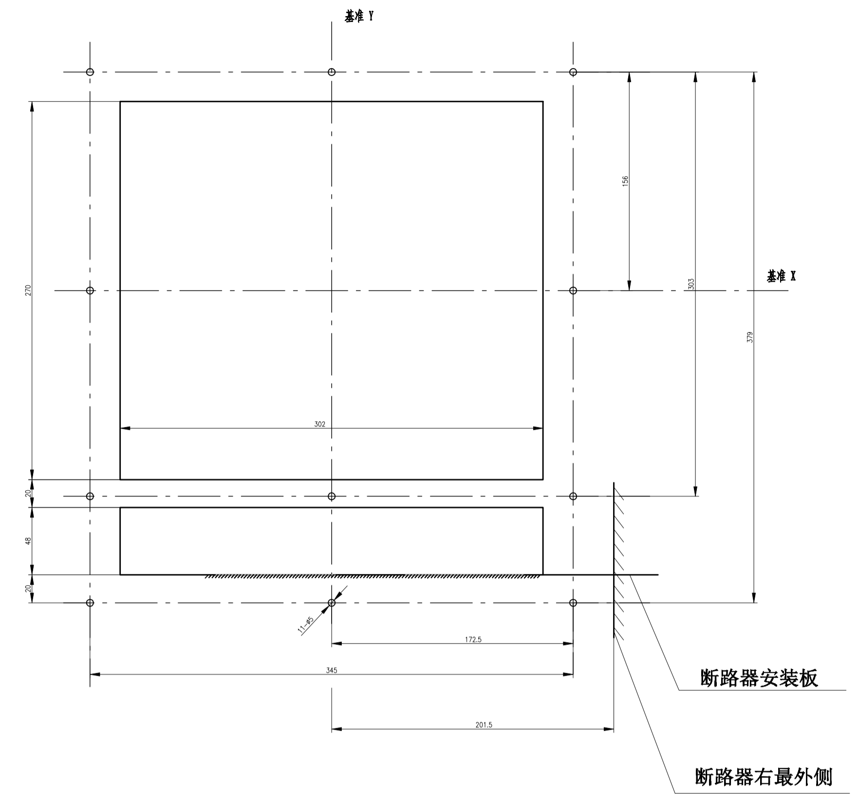
面板开孔
