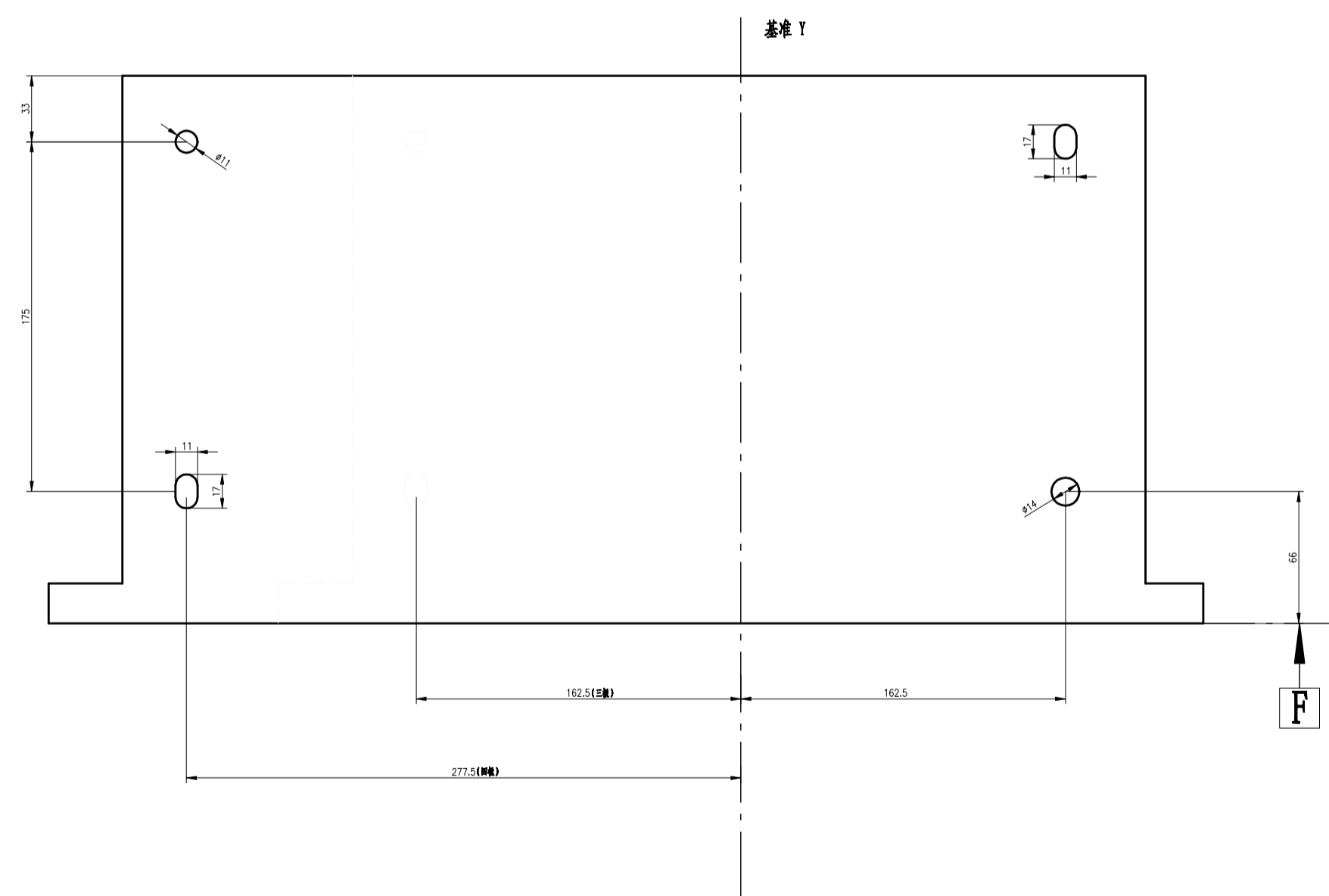
底面外形尺寸及安装孔距示意图
