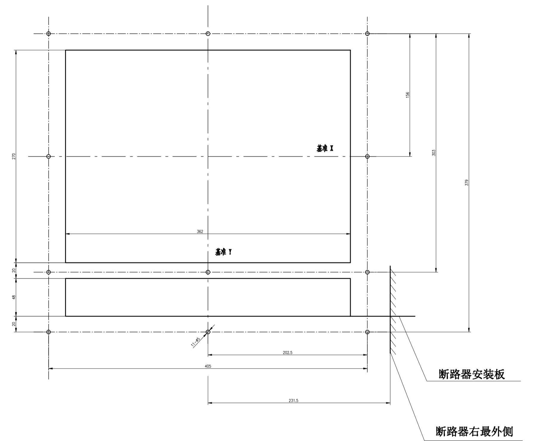
面板开孔
