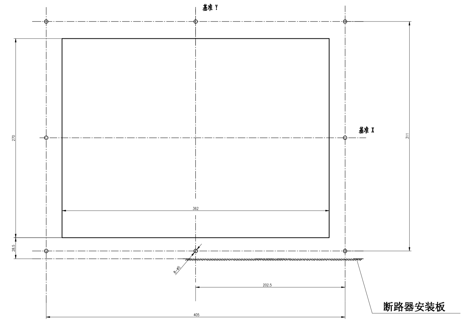
面板开孔
