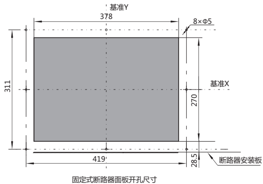
面板开孔尺寸
